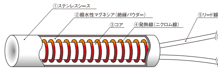
【カートリッジヒーターの基本構造図】
