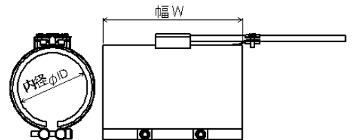
BH-5 型 (リード線出型トンボ+カバー付)
