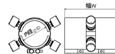
BH-7 型 (2 P 両端子型)
