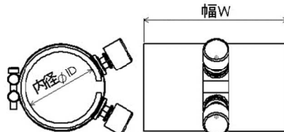
BH-2 型 (1 P 両端子型)
