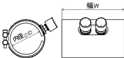
BH-1 型 (1 P 片端子型)
