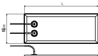
P H - 6 型 (リード片出型)
