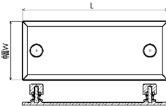
P H - 2 型 (両端子型)
