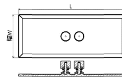
P H - 4 型 (端子中央 B 型)
